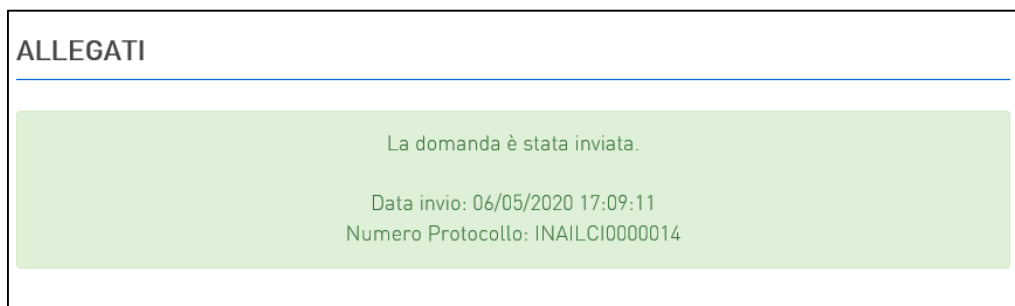
Figura 38: Domanda inviata
